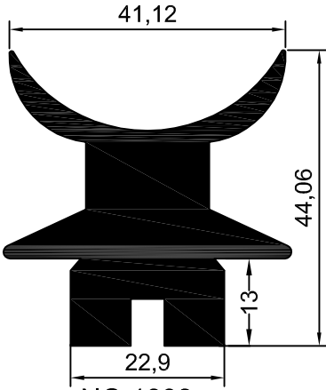
NO:1893 AY BAĞLANTI 2,542kg/m
