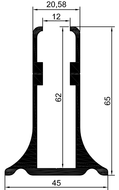
NO:2043 ETEK PROFİLİ 1,363 kg/m
