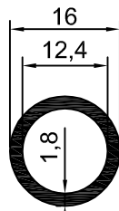
1.8mm 16'LİK EMNİYET ŞERİDİ BORUSU 0,424 kg/m
