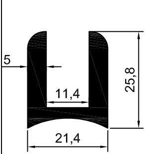
NO:2171 KANALSIZ CAM TUTAMAĞI 0,742 kg/m
