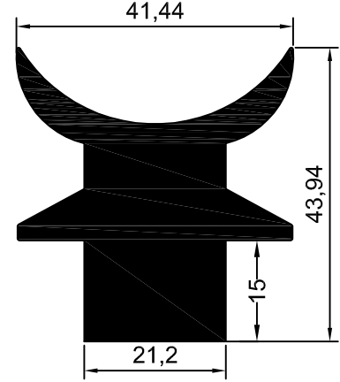
NO:1840 AY BAĞLANTI 2,511kg/m
