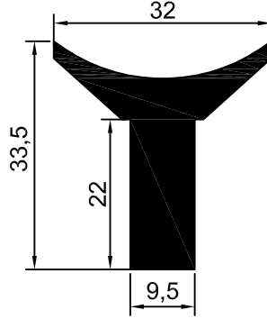
NO:1609 AY BAĞLANTI 0,994kg/m
