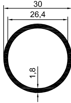
1.8mm 30'luk BORU 0,432 kg/m
