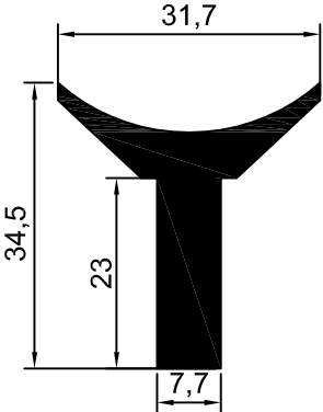
NO:1839 AY BAĞLANTI 0,857kg/m
