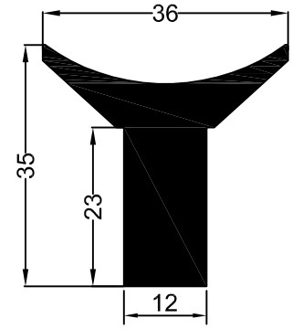
NO:2802 AY BAĞLANTI 1,050kg/m
