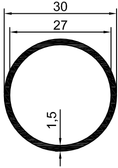
1.5mm 30'luk BORU 0,364 kg/m
