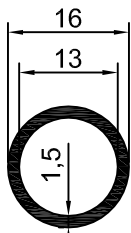
1.5mm 16'lık EMNİYET ŞERİDİ BORUSU 0,185 kg/m
