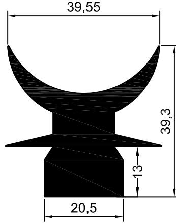
NO:1894 AY BAĞLANTI 2,542kg/m
