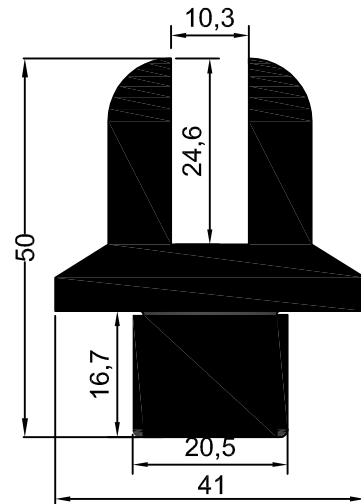
NO:1845 AY BAĞLANTI ALTI 2,717kg/m
